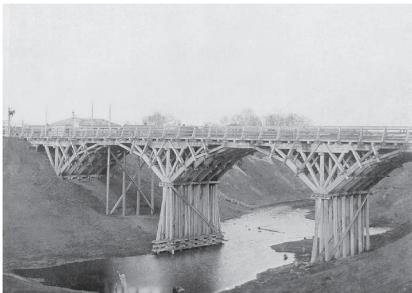
Мост на Стриковской улице. Построен в 1885 г. (фото около 1900 г.)
