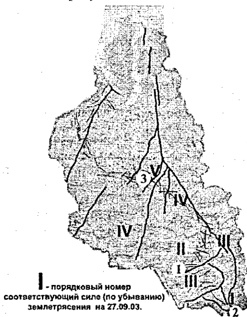
Рис. 1. Дифференциация территории Западной Сибири по силе землетрясения 27.09.03, и показана сеть тектонических разломов фундамента Западно-Сибирской молодой эпипалеозойской плиты
