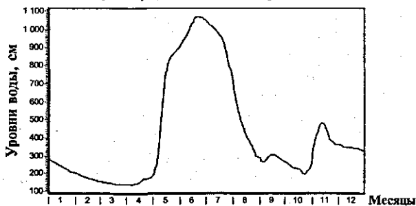
Рис. 1. Водомерный график р. Обь
