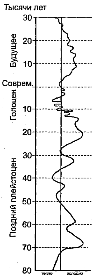
Рисунок 2. Усредненная кривая палеоклиматической и прогнозной температур для территории Западной Сибири.
