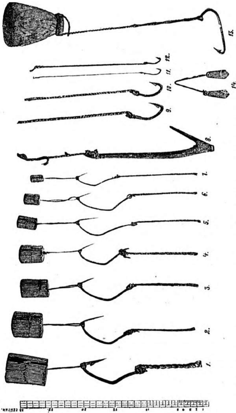
Различные крючковыя снасти: 1—5. Осетровые самоловы. 6—7. Стерляжи самоловы. 8. Деревянный крючокъ для лова налима. 9—10. Осетровые переметы. 11—12. Стерляжи переметы. 13. Озерная удочка. 14. Двѣ блесны.
