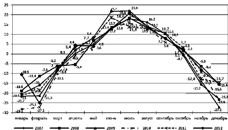
Рис. 8. График среднемесячной температуры воздуха ( ^{\circ}\text{C} ) г. Нижневартовска (2007-2012 гг) [13]
