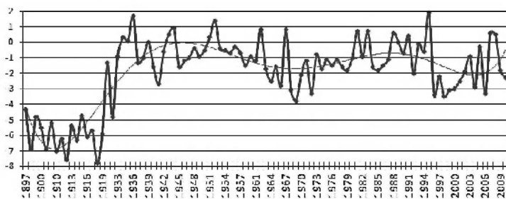
Рис. 4. График среднегодовой температуры воздуха (°C) г. Ханты-Мансийска (1897- 2010 гг.) [7]
