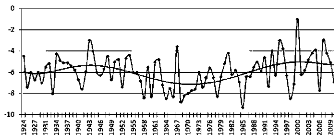
Рис. 2. График среднегодовой температуры воздуха ( ^{\circ}\text{C} ) г. Салехарда (1924 - 2010 гг.) [7]
