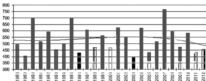
Рис. 7. Годовое количество атмосферных осадков (мм) г. Нижневартовска (1988 - 2011 гг.) [13]
