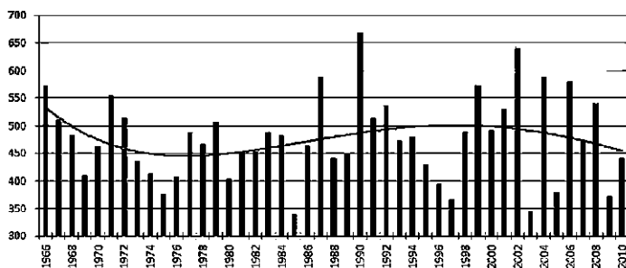
Рис. 11. Годовое количество атмосферных осадков (мм) г. Тюмени (1966 - 2010 гг.) [7]
