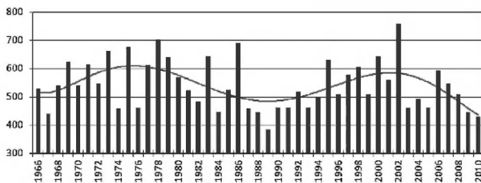
Рис. 5. Годовое количество атмосферных осадков (мм) г. Ханты-Мансийска (1966 - 2010 гг.) [7]
