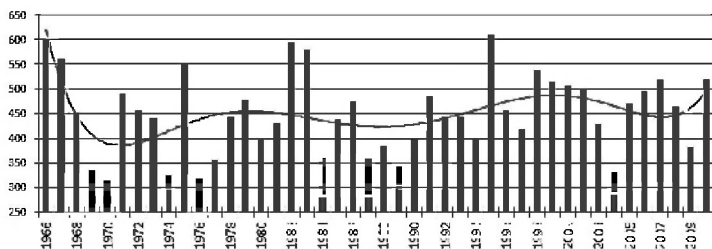
Рис. 3. Годовое количество атмосферных осадков (мм) г. Салехарда (1966 - 2010 гг.) [7]
