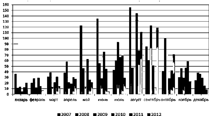
Рис. 9. Количество атмосферных осадков за месяц (мм) в г. Нижневартовске (2007-2012 гг.) [13]
