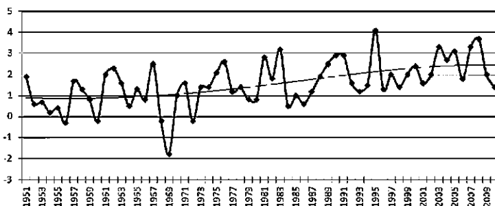
Рис. 10. График среднегодовой температуры воздуха (°С) г. Тюмени (1951 - 2010 гг.) [7]
