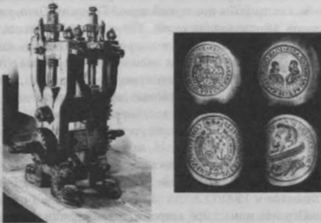
Рис. 5. Вальцевальный станок со сменными штампелями.
