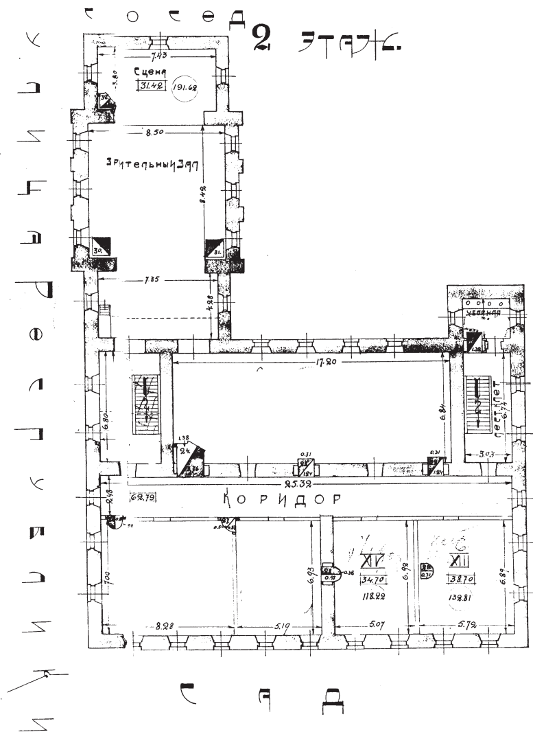
ПЛАН ВТОРОГО ЭТАЖА. 1930 г.
