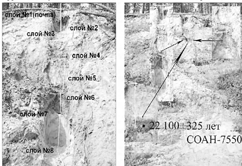
Рис. 2. Геологический разрез
