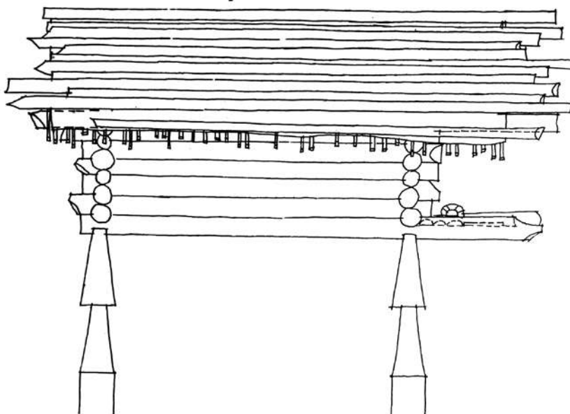
Вид с запада М1:20
