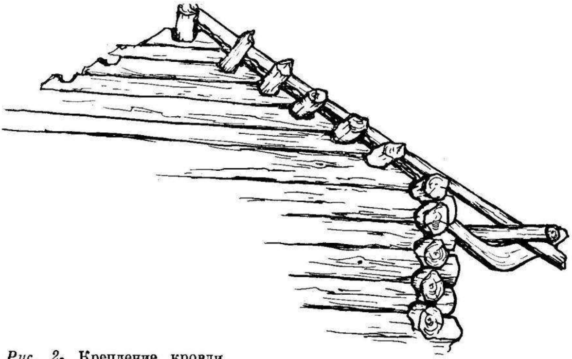
Рис. 2. Крепление кровли.
